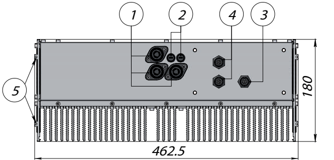
Модуль силовой (вид спереди)
