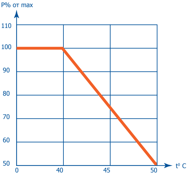
Рекомендуемая нагрузочная способность выпрямителя от температуры окружающей среды
