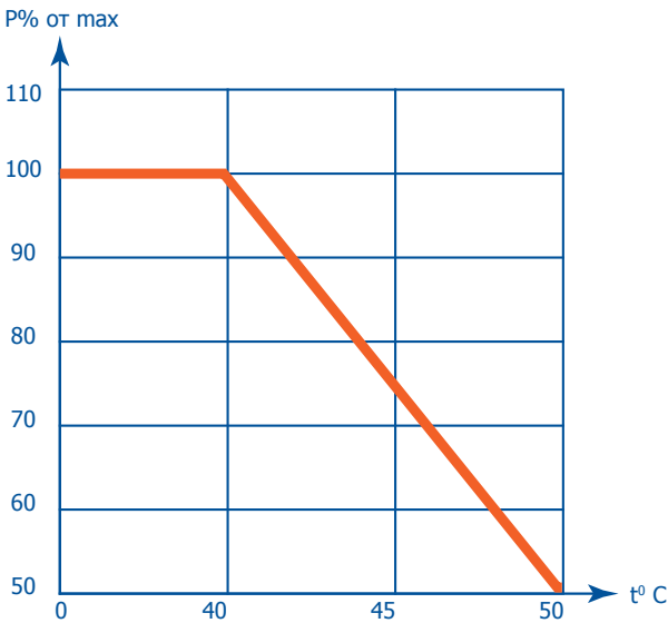
Рекомендуемая нагрузочная способность выпрямителя от температуры окружающей среды
